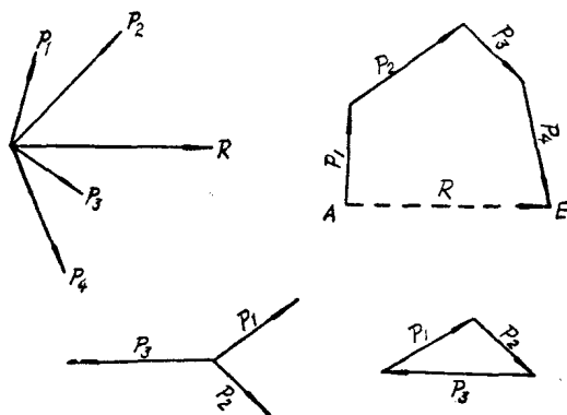
图 1—7 作用于一点的几个力的合成
