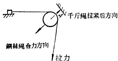
图 1—10 转向滑车的力的平衡
