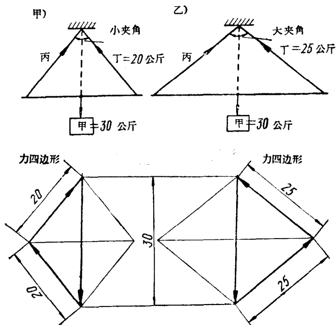
图 1—8 千斤绳夹角与受力大小
