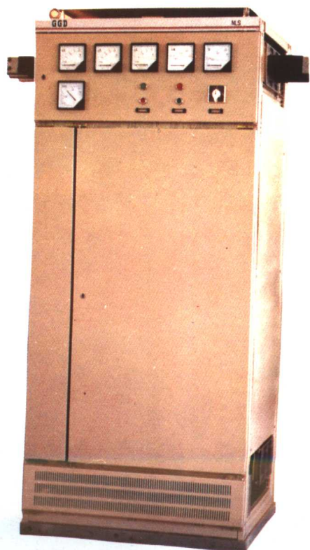
GGD 低壓配電屏
