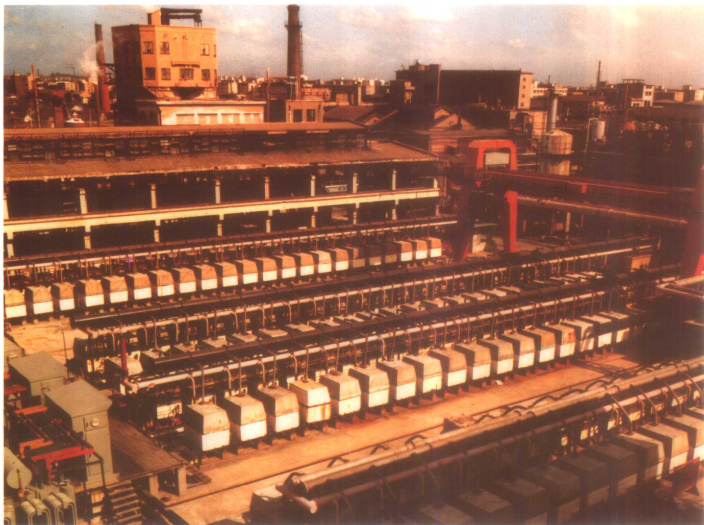
上海天原化工厂金属阳极电解槽一角
