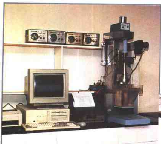
▲ 实验室电化学控制浮选系统
