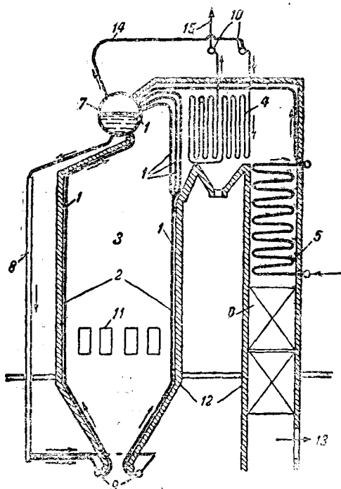
圖 3-2. 現代大型鍋爐圖
