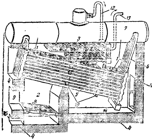
圖 3-1. 簡單小型鍋爐設備圖
