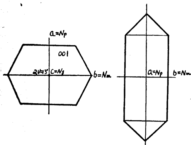
图 1-6 \alpha 型半水石膏的晶形
