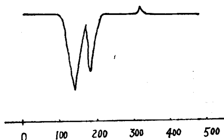
图 1-4 二水石膏的差热曲线
