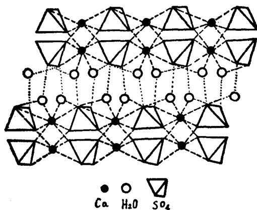
图 1-1 二水石膏的结晶结构
