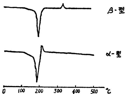
图 1-7 \alpha 型与 \beta 型半水石膏的差热曲线
