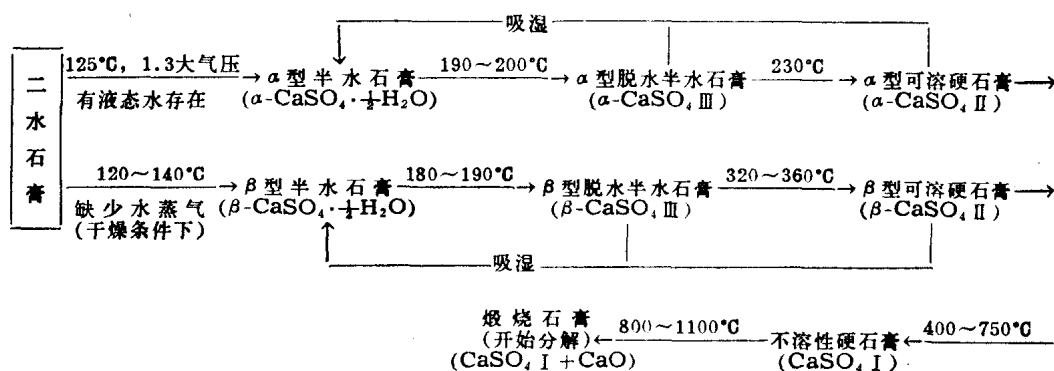
图 1-3 石膏的变种
