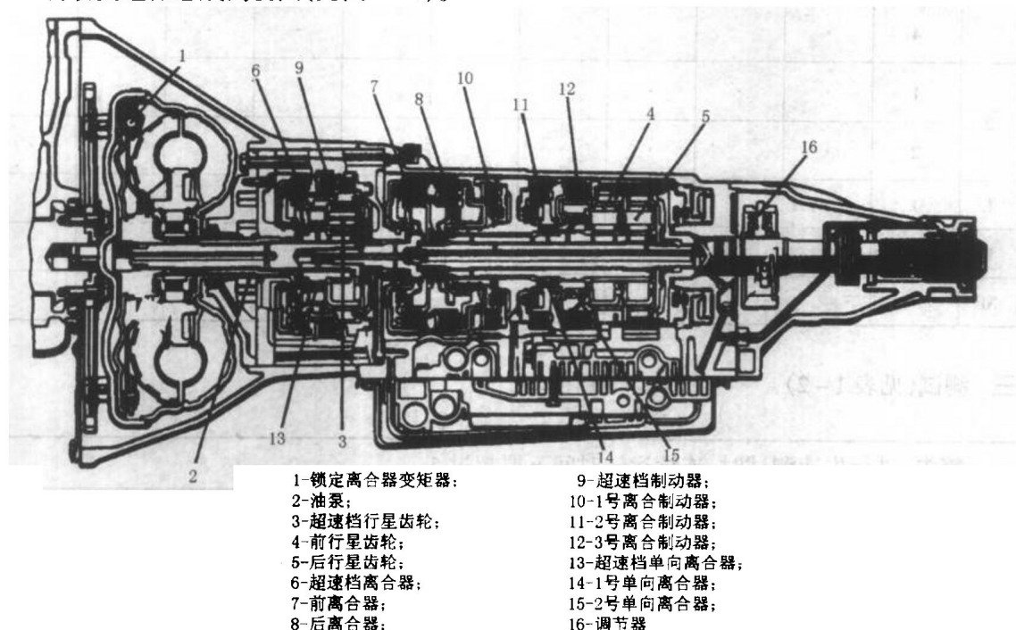
图 1-1 自动变速器总成剖视图
