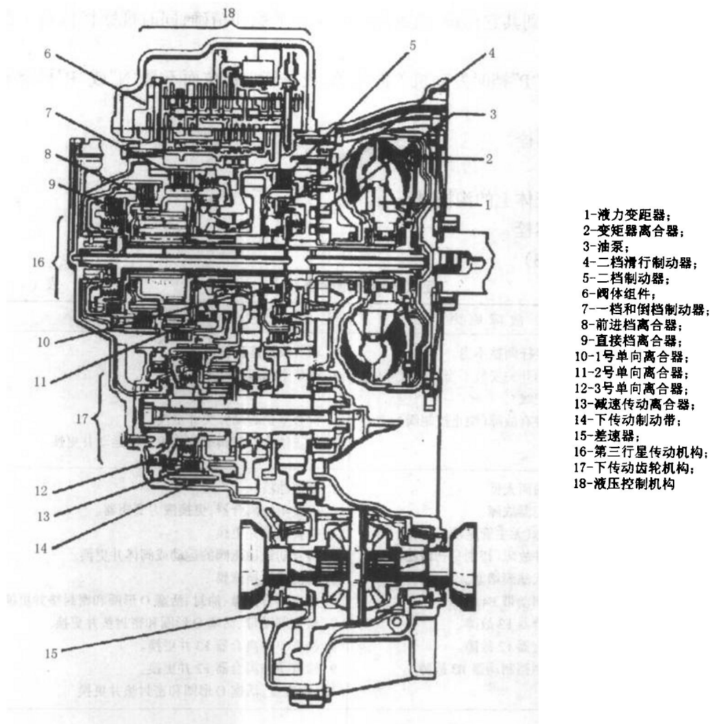
图 1-12 变速器部件剖视图
