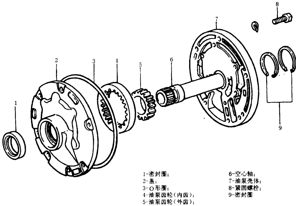
图 1-4 油泵分解图
