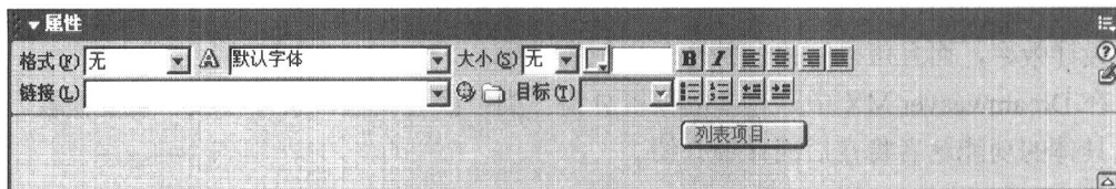
图 1-15 “属性”面板
