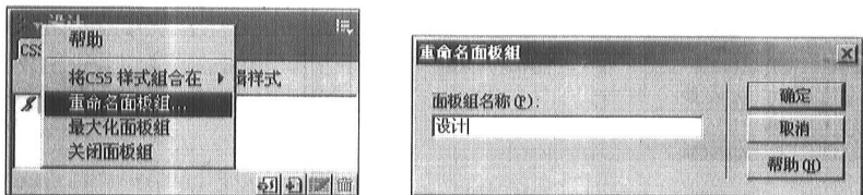
图 1-12 面板改名
