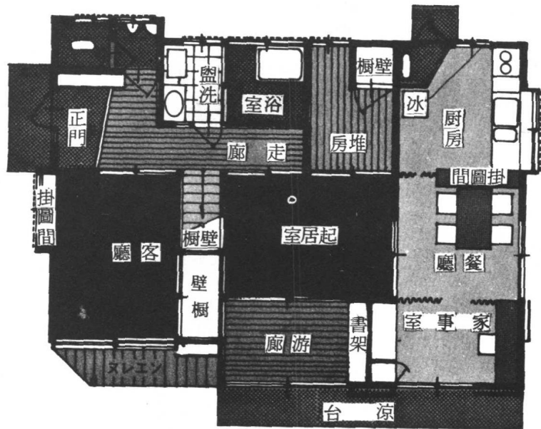
面平樓一
