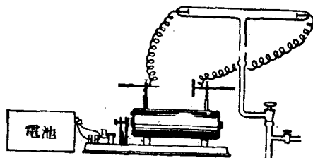
圖 1 真空抽氣機
