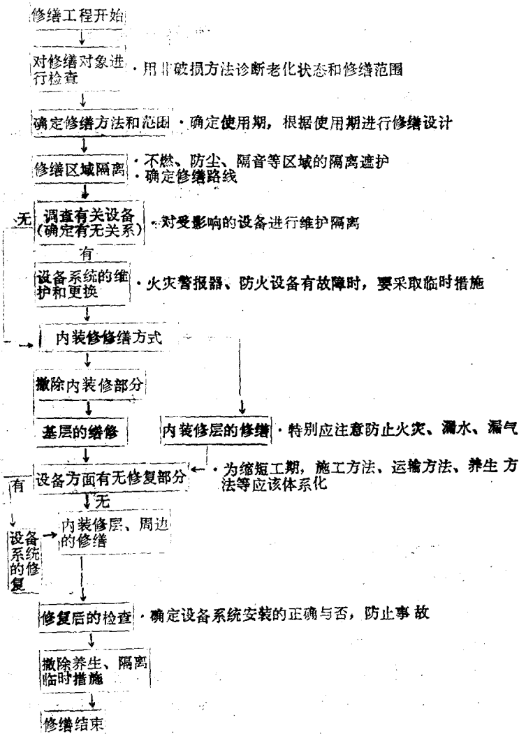
图1-1 室内修缮工程程序
