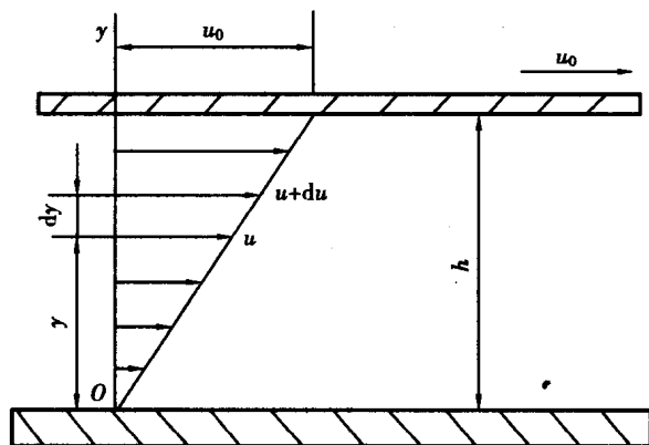
图 2.1 液体粘性示意图
