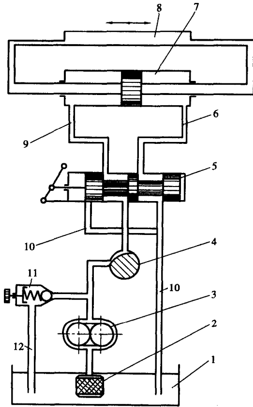
图 1.2 液压传动系统结构原理图
