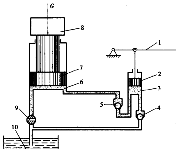
图 1.1 液压千斤顶原理示意图
