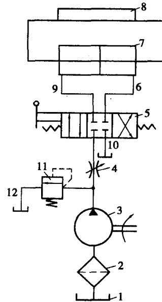
图 1.3 液压传动系统工作原理图
