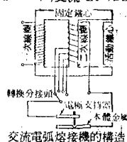
交流電弧熔接機的構造
