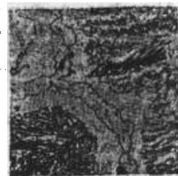
異常組織 × 500
