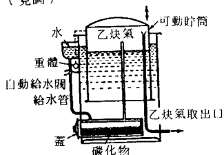
乙炔發生器 (本體構造)
