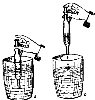
第162圖 吸管
