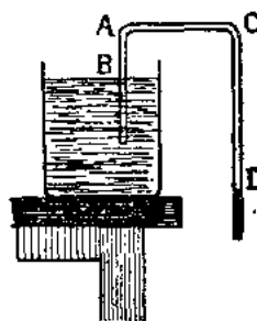
第164圖 虹吸管
