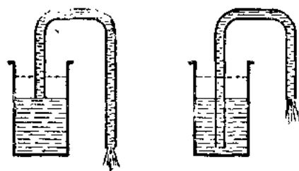
第 166 圖 虹吸管上出水的一瞬間
