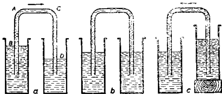
第 165 圖 虹吸管實驗
