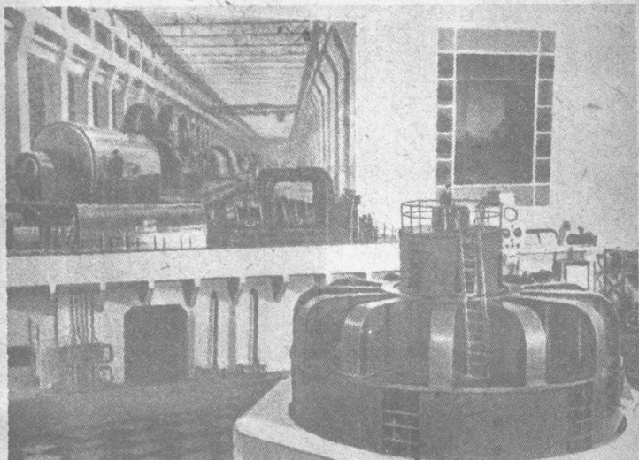
蘇聯強大的渦輪發動機和水力發電機
