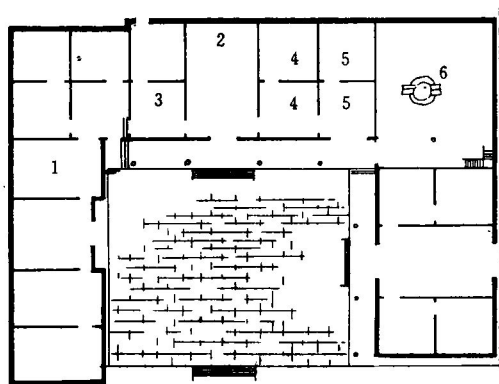
图 7-2 邓小平旧居平面示意
