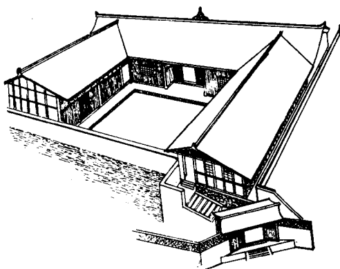
图 7-6 丁佑君故居透视
