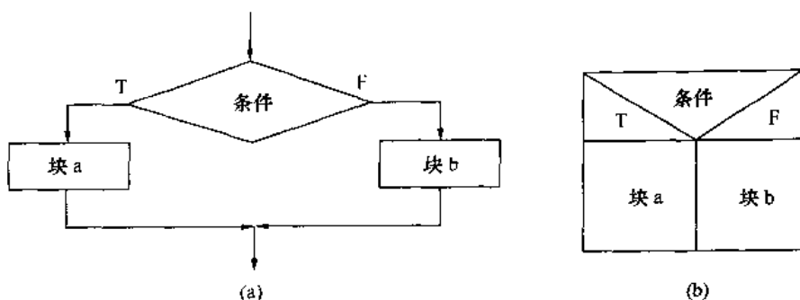
图 1-4 选择结构流程图
