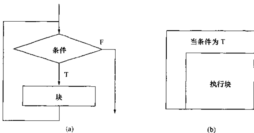
图 1-5 循环结构流程图
