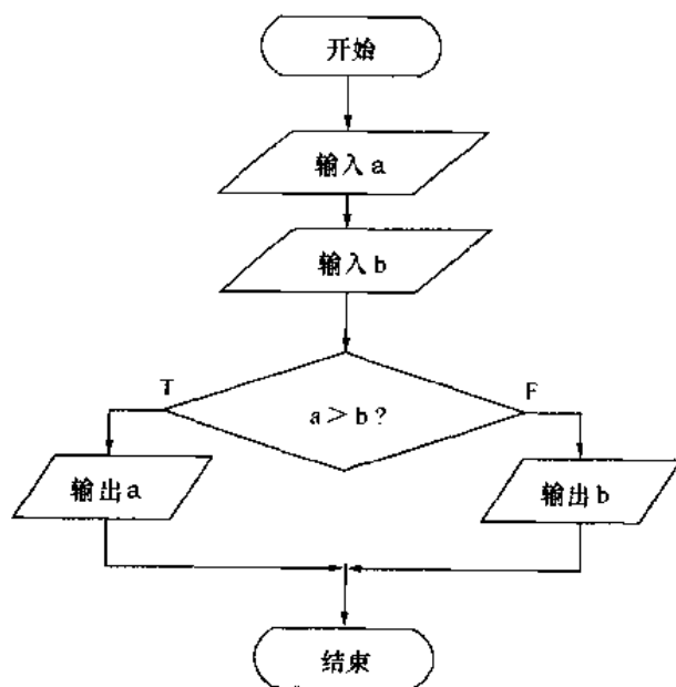
图 1-2 例 1-1 算法的流程图
