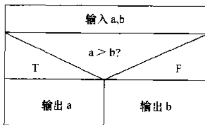
图 1-6 例 1-2 算法的 N-S 流程图
