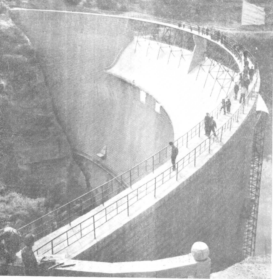
四川省长沙坝水库的砌石拱坝
