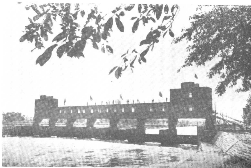
都江堰灌区新建的 人民渠进口节制閘
