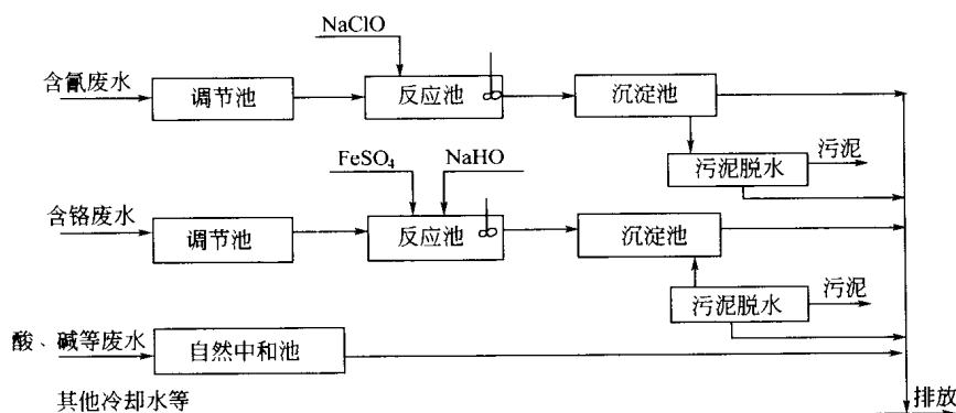
图 1-1 传统的电镀废水处理流程
