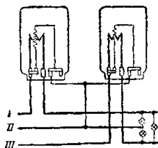
圖 1-7. 三相三線制電力網 中用兩隻單相電度表計算 電能的接線圖
