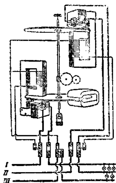
圖 1-9. 計算三線制電力網中電能的三相電度表的構造圖和接線圖
