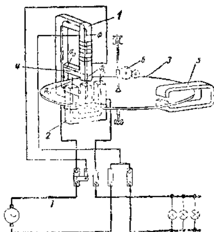
圖 1-1. 交流電度表的構造示意圖
