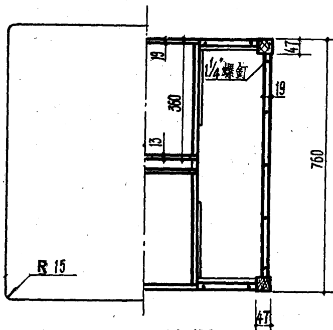
二剖面图
