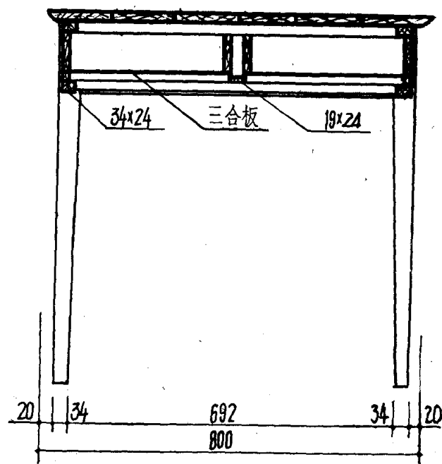
一剖面图
