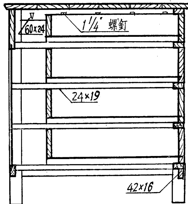
二剖面图
