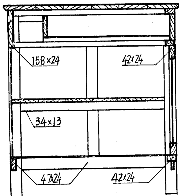
一剖面图
