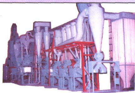
6FYDT-20 型玉米综合利用成套设备
