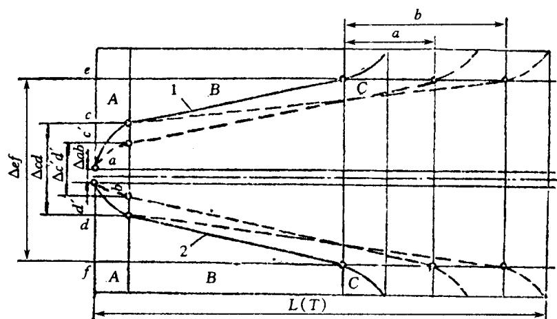
图 0-1 配合零件的磨损规律
