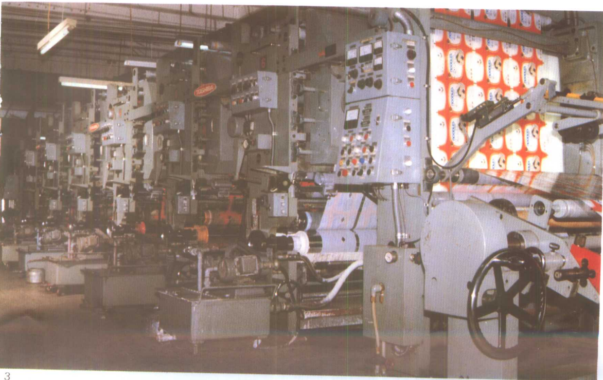
3 上海人民塑料印刷厂六色轮转印刷机
