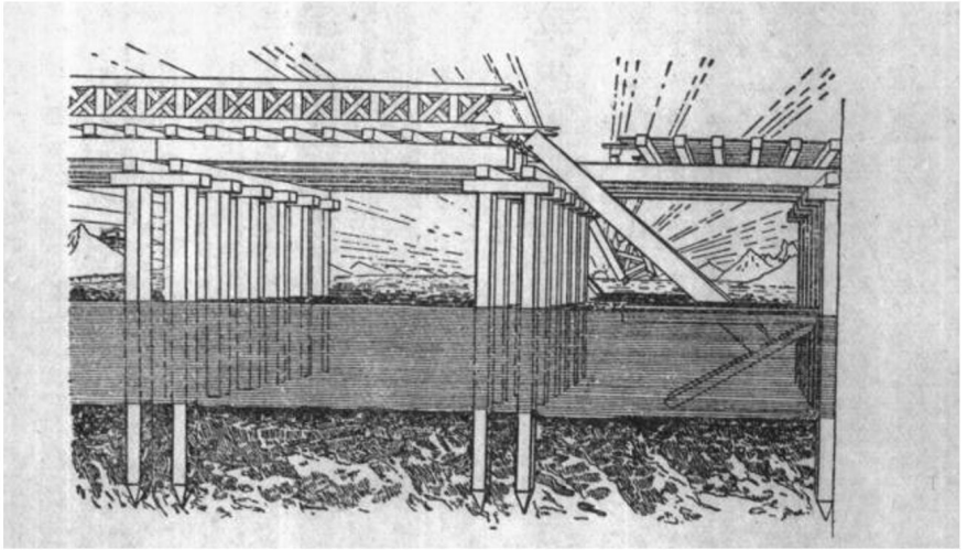
圖 5. 羅馬跨過底勃爾河的梁式橋梁，築成於公元前 630 年左右。
