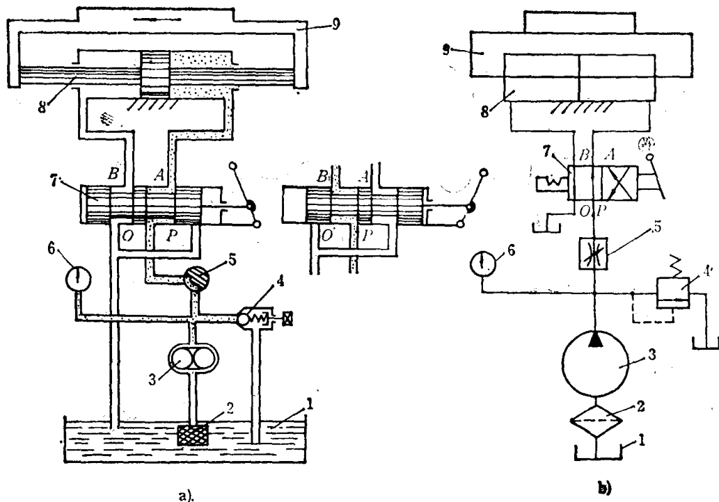
图 1-2 简化的磨床工作台液压系统图
