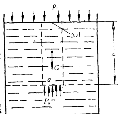
图 1-5 深度为 h 处的液体的压力
