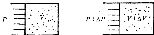
图 1-3 压力升高时,油液体积的变化
