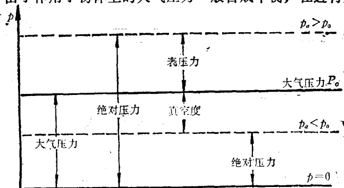
图 1-6 绝对压力、相对压力和真空度的关系
