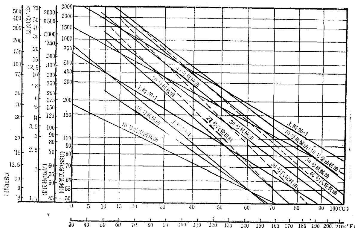
图 1-4 国产油粘温图
