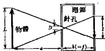
圖 2 針孔的 F 值。
