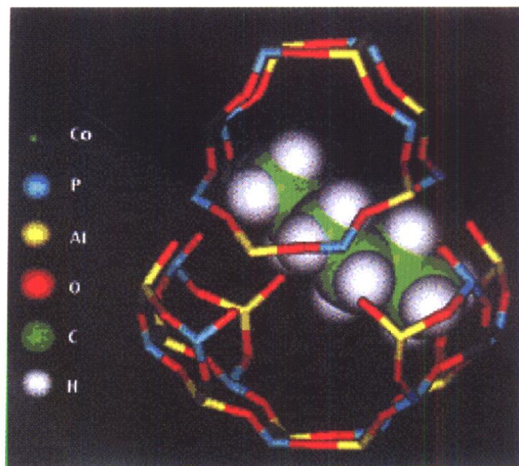
彩图 7 含钴磷酸铝沸石催化氧化 正己烷直接得到己二酸
