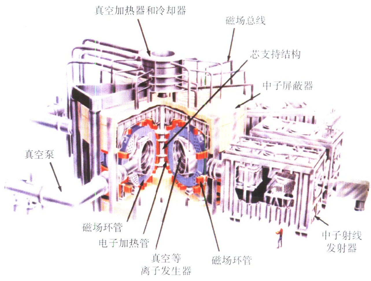
彩图 9 可控聚变反应堆
