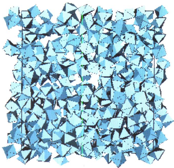
彩图 4 氟化物玻璃结构模型
