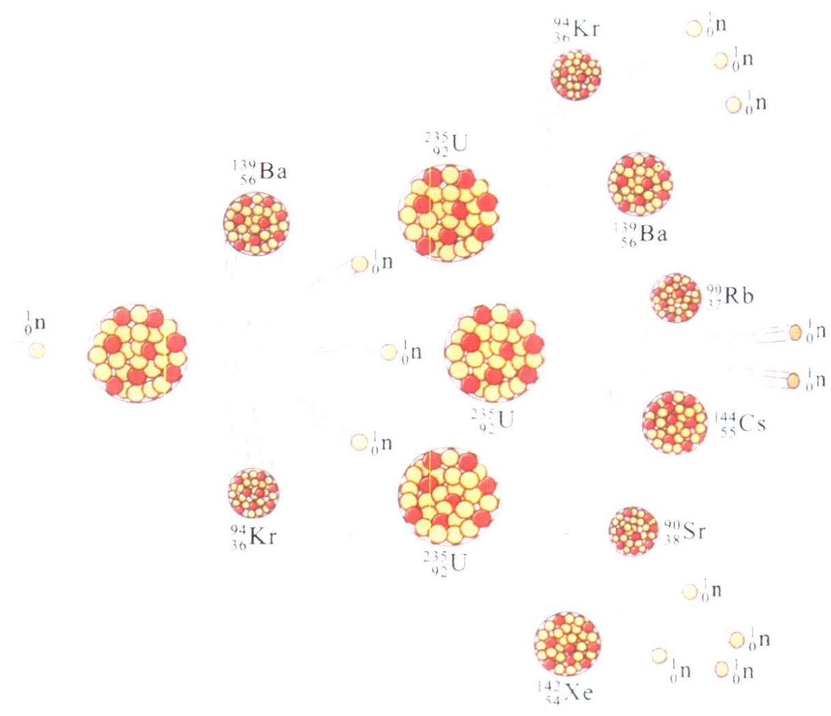
彩图 8 链式裂变
