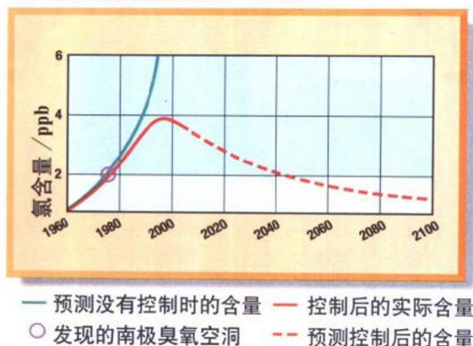
大气层中氯的含量(1960~2100)
