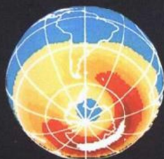
1979年 卫星图像 显示臭氧层变薄了
