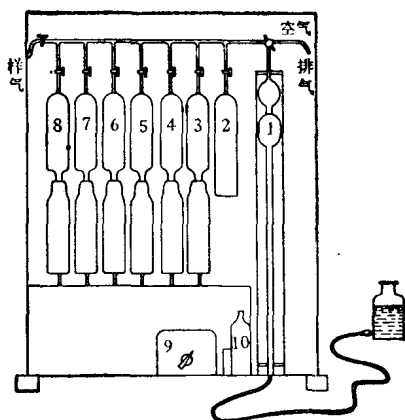
图1 奥氏体分析仪装置
