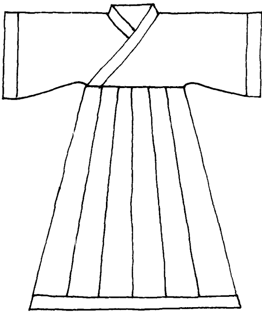
图1-4 深衣示意图
