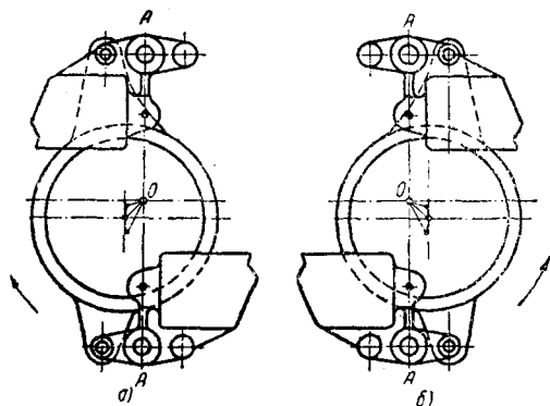
圖4. II-25 機車平面調速器構造
