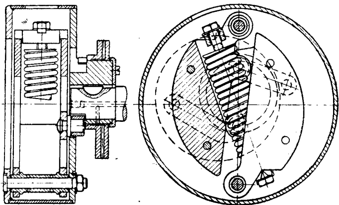
圖 6. ЦКТИ 小型汽力裝置平面離心調速器
