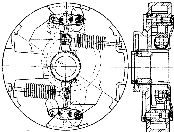
圖 5. II-25 型機車調速器
