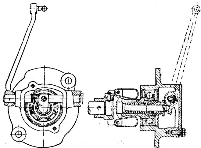
圖 3. Д-3 汽油機離心調速器
