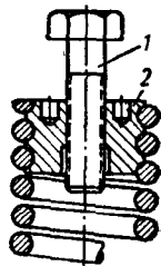
圖 7. ЦКТИ 調速器和彈簧的 聯結
