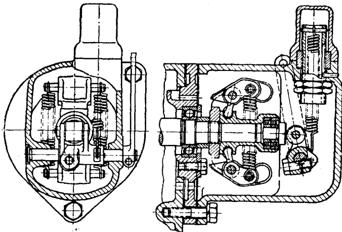
圖2. CXT3-HATI 拖拉機原機離心調速器
