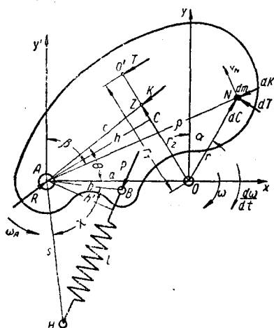
圖 8. 作用在平面離心調速器離心重量上的各種作用力構圖
