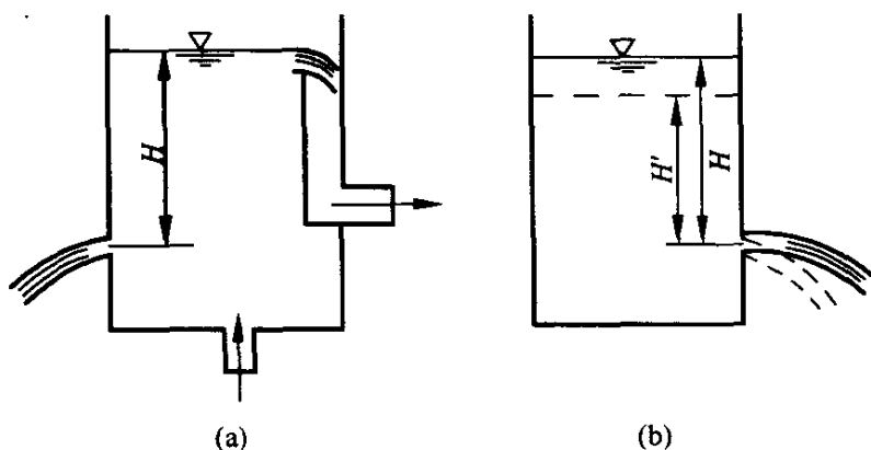
图 1.2 恒定流和非恒定流
