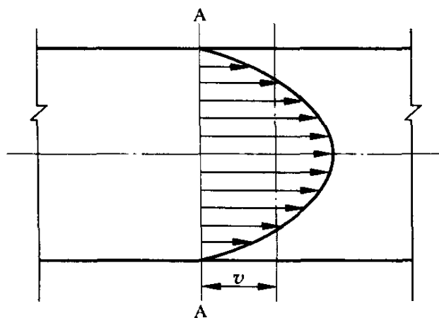
图 1.1 管道中流速分布
