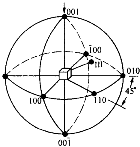
图 1-14 参考球与立方系球面投影
