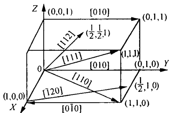
图 1-10 正交系中一些晶向指数
