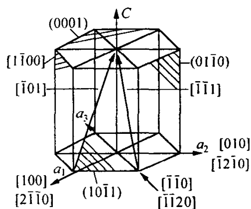
图 1-12 六方系的一些晶面与晶向指数
