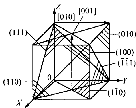
图 1-11 立方系常用晶面指数
