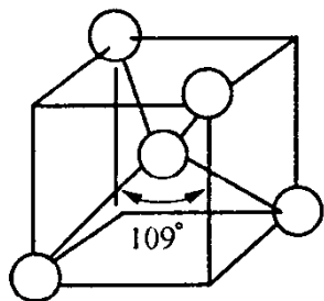
图 1-1 Si 形成的四面体
