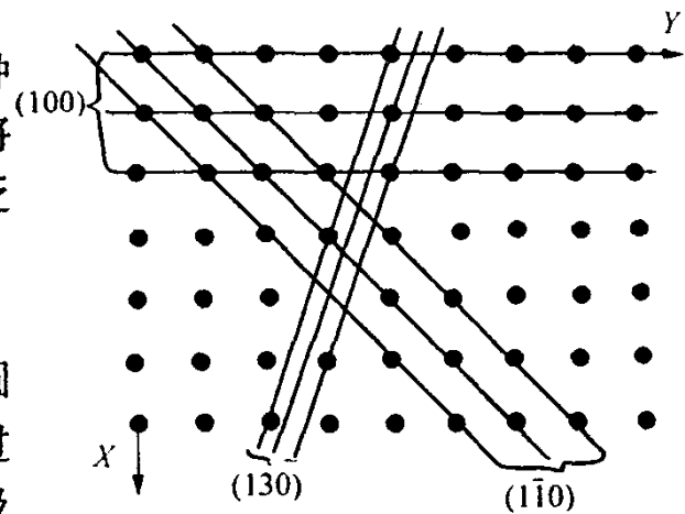
图 1-13 晶面间距
