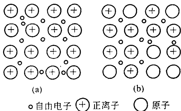
图 1-3 金属键模型
