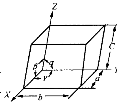
图 1-8 晶胞、晶轴及点阵参数
