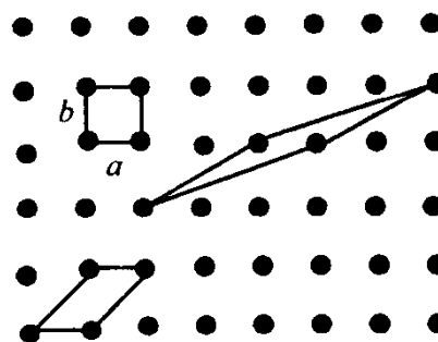
图 1-7 在点阵中选取晶胞
