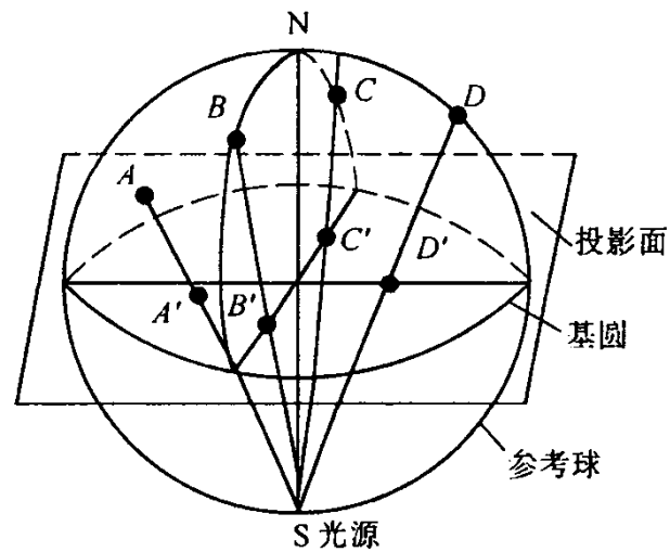
图 1-15 极射赤面投影
