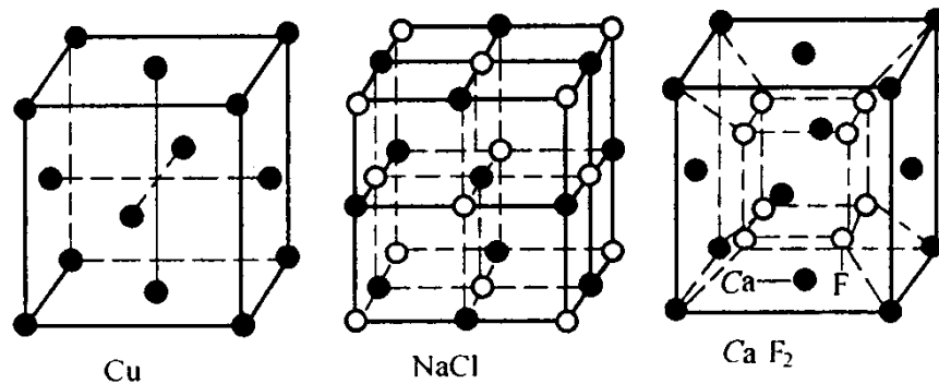
图 1-9 具有相同点阵的晶体结构
