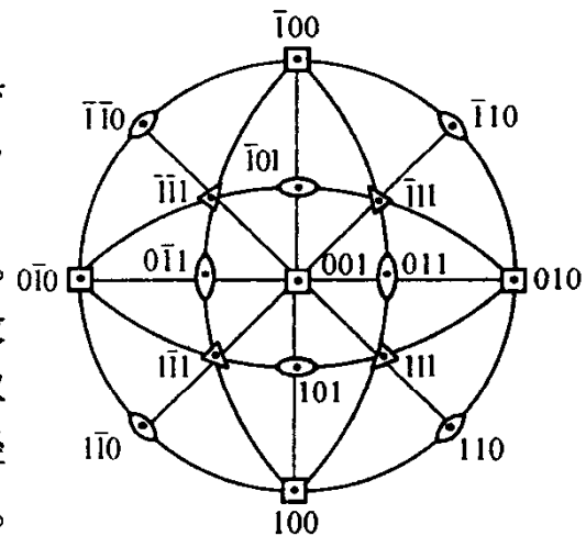
图 1-16 立方系(001)标准投影图
