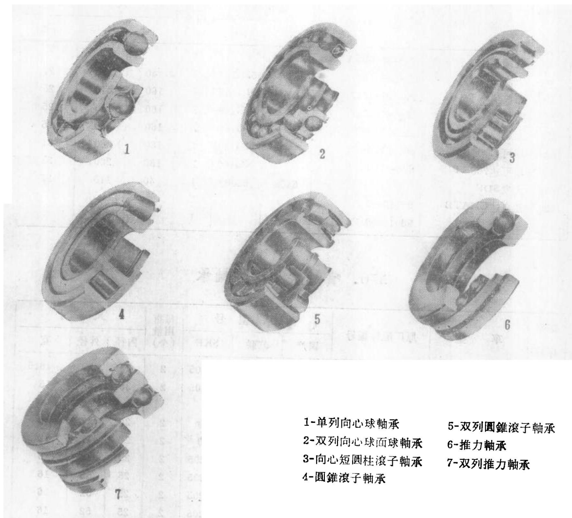
图436 各型轴承
