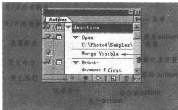
图 1.3 Action 调色板
