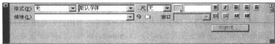
图 1-2-1 属性栏
