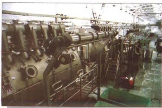
德国TS大容量高温高压染色机
