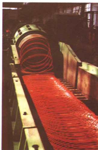
高速线材成品线
