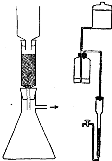
图 10 加压裝置
