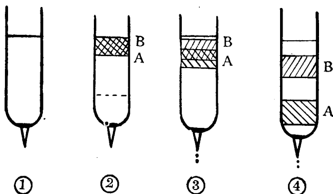
图1 二元混合物之吸附层离法
