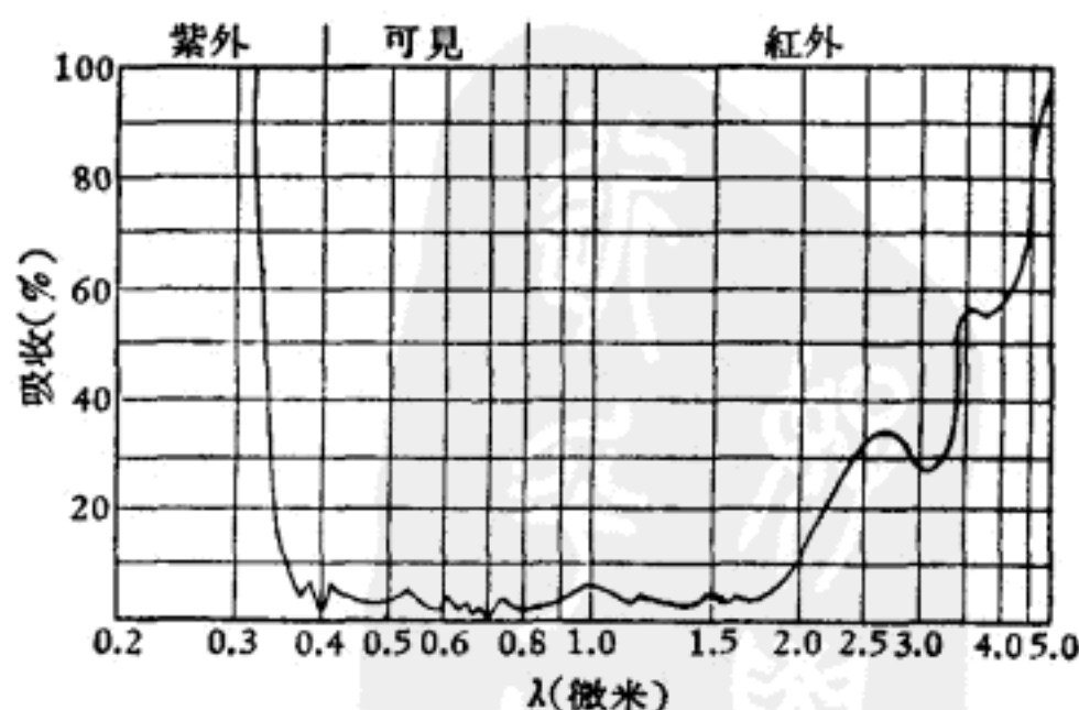
图 1 一种冕牌玻璃的吸收曲线
