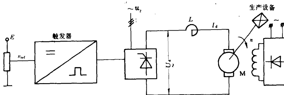
图 1-4 V-M 系统原理图
