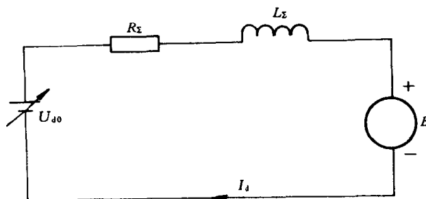
图 1-5 V-M 系统等值电路
