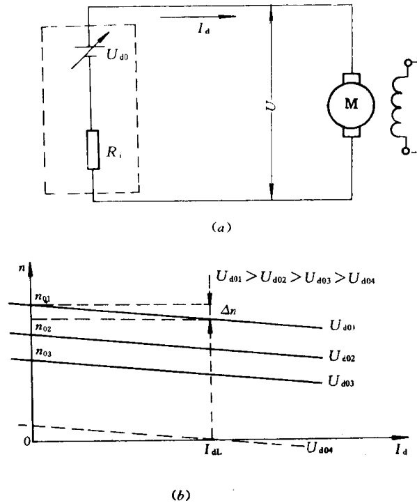
图 1-1 变电枢电压调速系统 (a) 电路; (b) 机械特性
