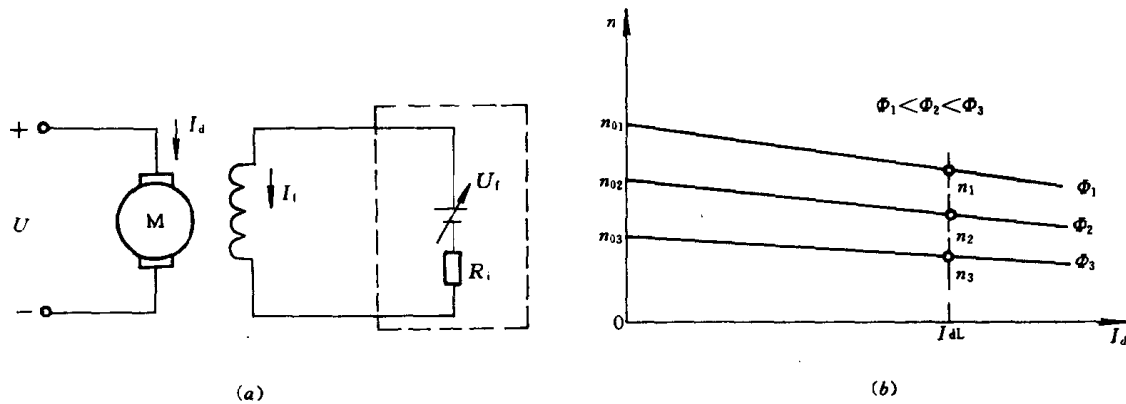
图 1-2 磁场调节调速系统 (a)原理图;(b)机械特性
