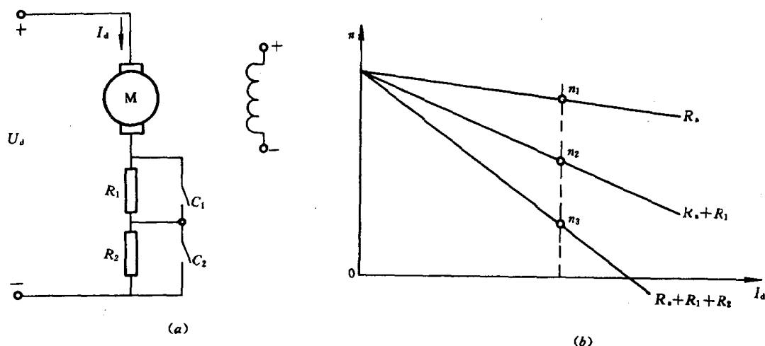
图 1-3 改变电枢电阻调速系统 (a)电路;(b)机械特性
