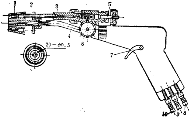
图7-3-3 塑料喷枪
