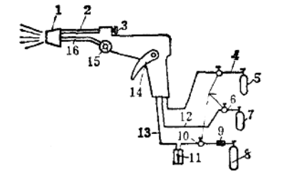
图7-3-2 火焰喷涂设备系统图
