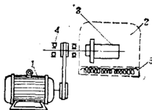
图7-2-3 离心浇注装置示意图 1—电机 2—铸型 3—铸造尼龙件 4—离心装置 5—电加热器
