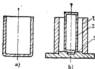
图7-2-2 铸型尼龙模具 a) 无芯棒体成型 b) 有芯筒成型 1—圆筒 2—芯子 3—底板
