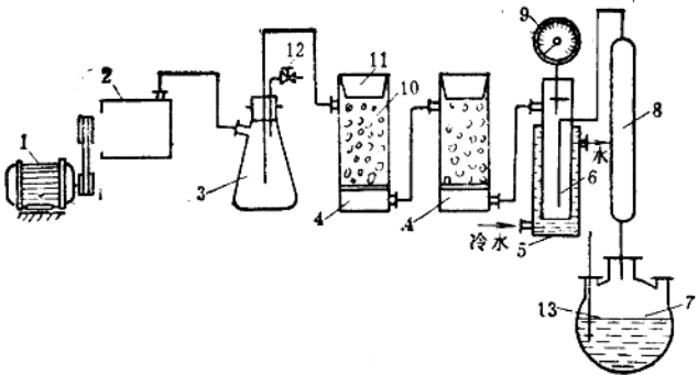
图7-2-1 铸型尼龙工艺流程示意图
