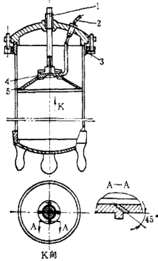
图7-3-4 飞扬式送粉桶
