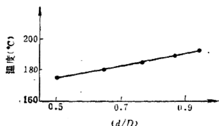
图7-2-4 聚合温度与 d/D 比值的关系
