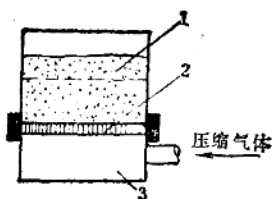
图7-3-1 沸腾床 1—沸腾室 2—多孔底 3—气室
