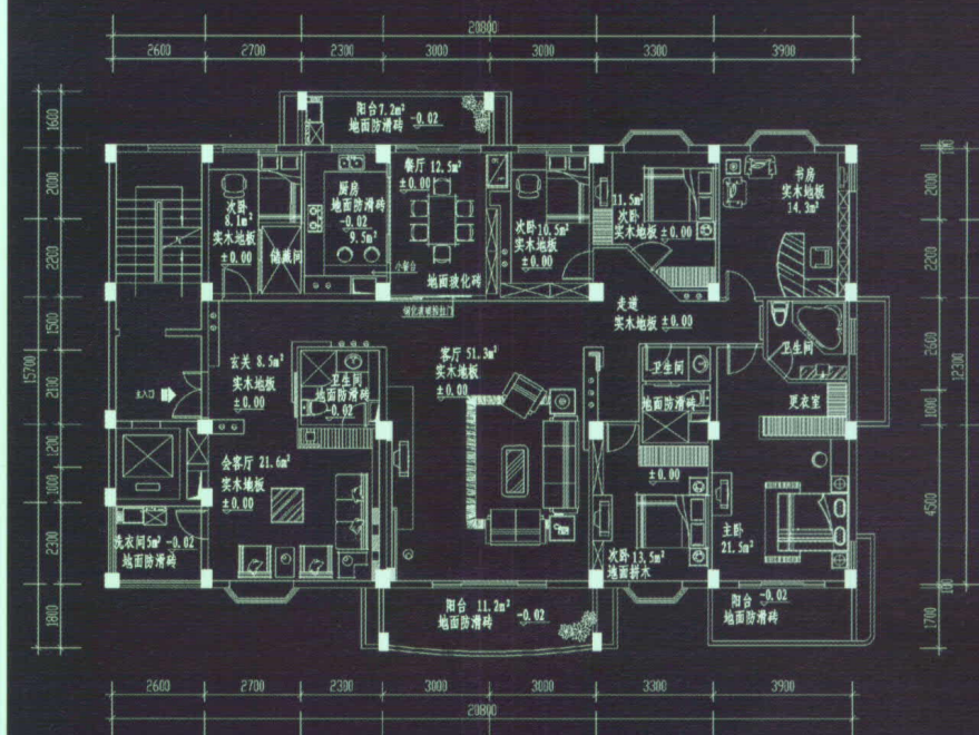
平面布置图
