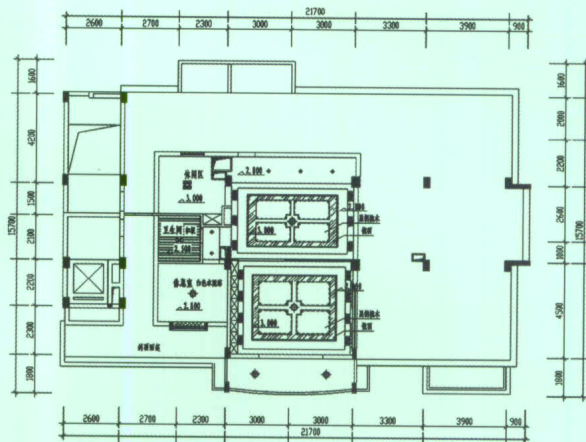
二层吊顶布置图
