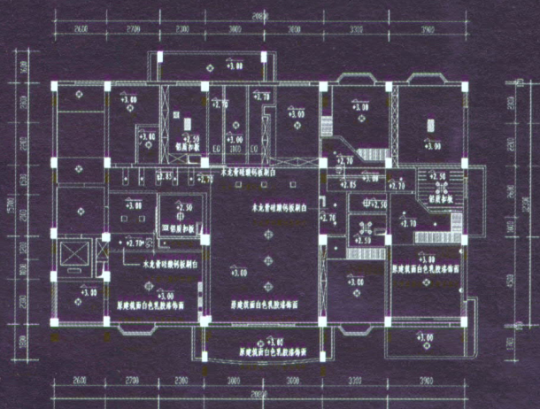
吊顶布置图
