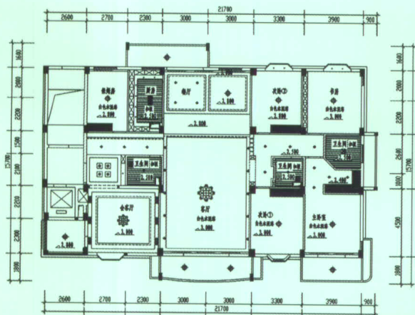
一层吊顶布置图
