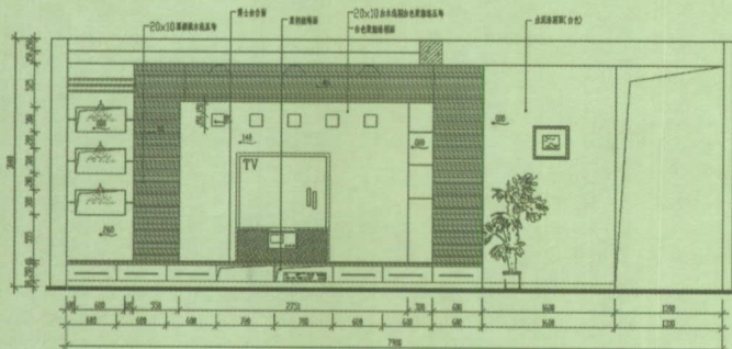
客厅电视柜立面图
