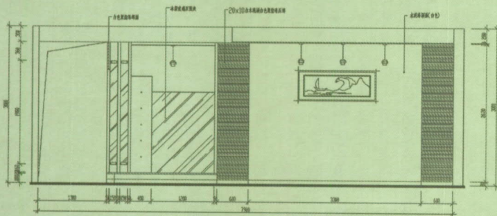
客厅沙发背景立面图
