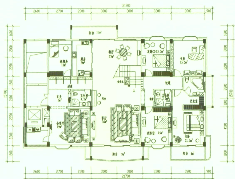
一层平面布置图
