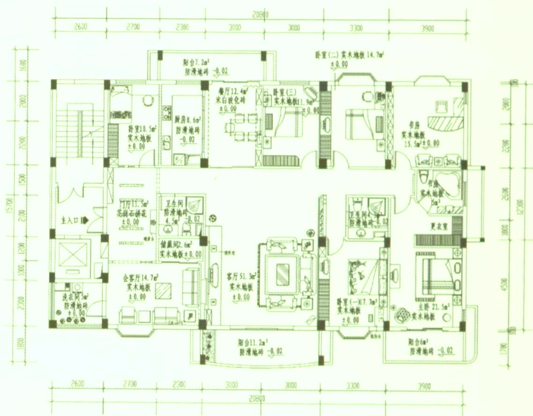
平面布置图
