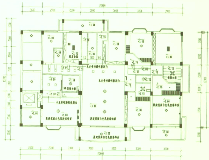
吊顶布置图
