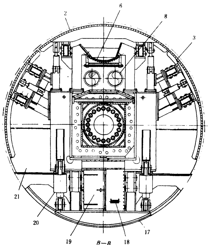
图 1—1(b) Jarva Mk27/8.8 之 B—B 剖视图
