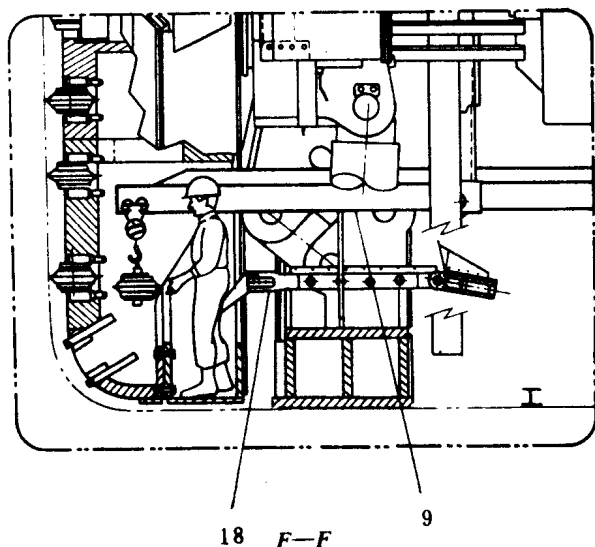
图 1—1(f) Jarva Mk27/8.8 之 F—F 剖视图
