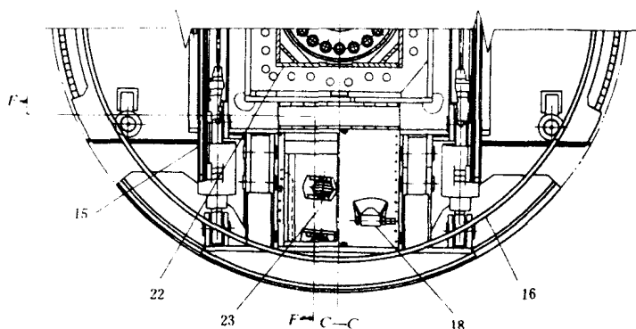
图 1-1(c) Jarva Mk27/8.8 之 C—C 剖视图
