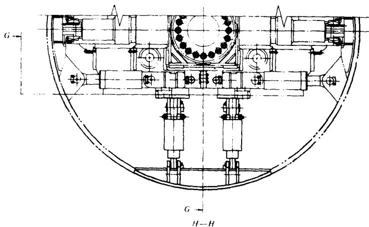
图 1-1(h) Jarva Mk27/8.8 之前支腿后视图
