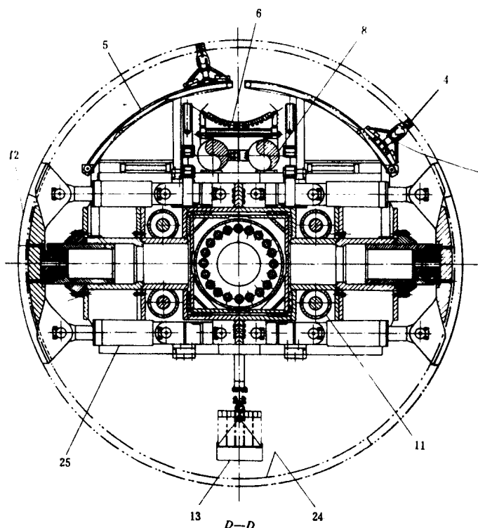
图 1—1( d ) Jarva Mk27/8.8 之 D—D 剖视图
