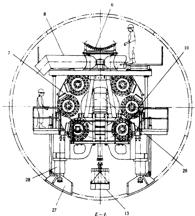
图 1—1(c) Jarva Mk27/8.8 之 E—E 剖视图
