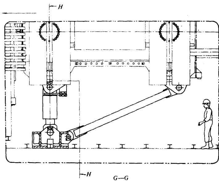
图 1-1(g) Jarva Mk27/8.8 可装可不装之前支腿(任选)
