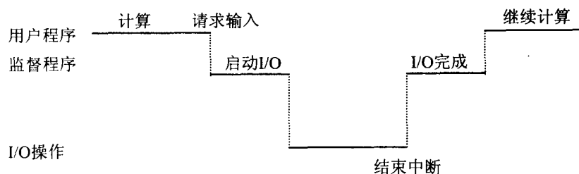
图 1.4 单道程序工作示例
