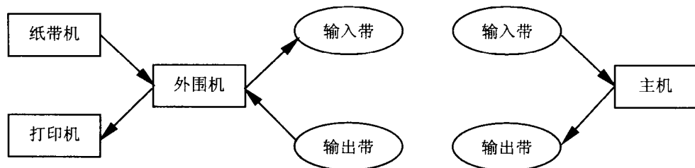
图 1.3 脱机输入输出方式
