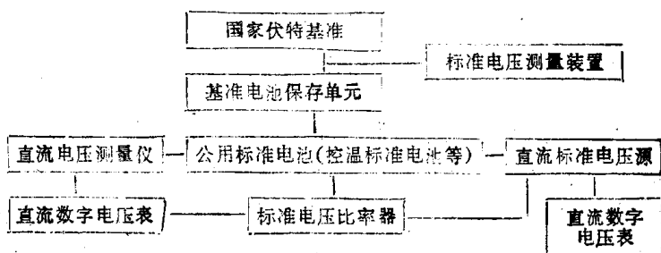
图1-1 直流标准电压的量值传递系统图
