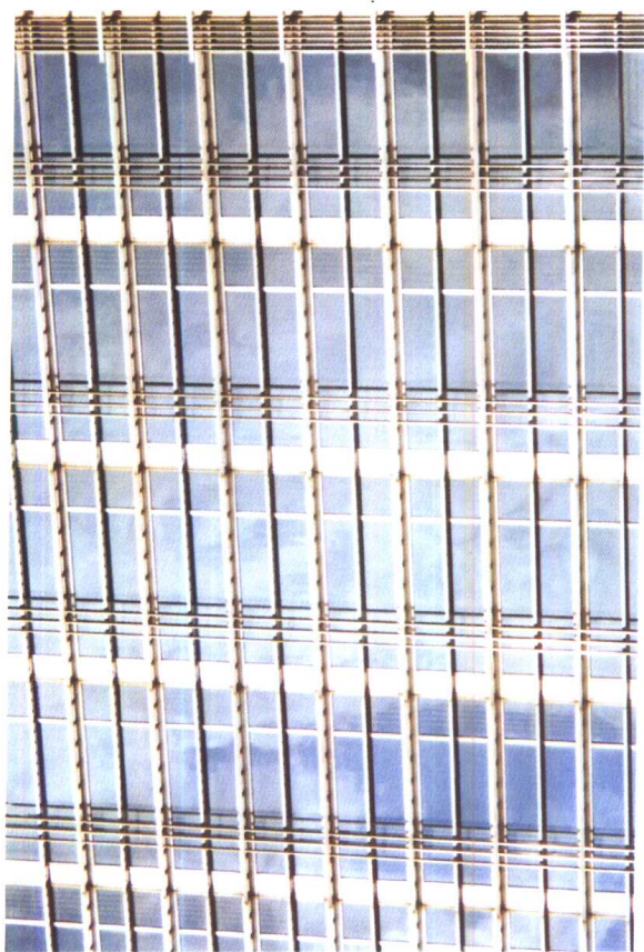
1.18 上海金茂大厦幕墙细部 (明框幕墙, 外面有不锈钢装饰)
