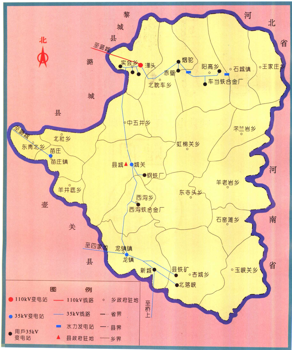
平顺县1996年地理主接线示意图
