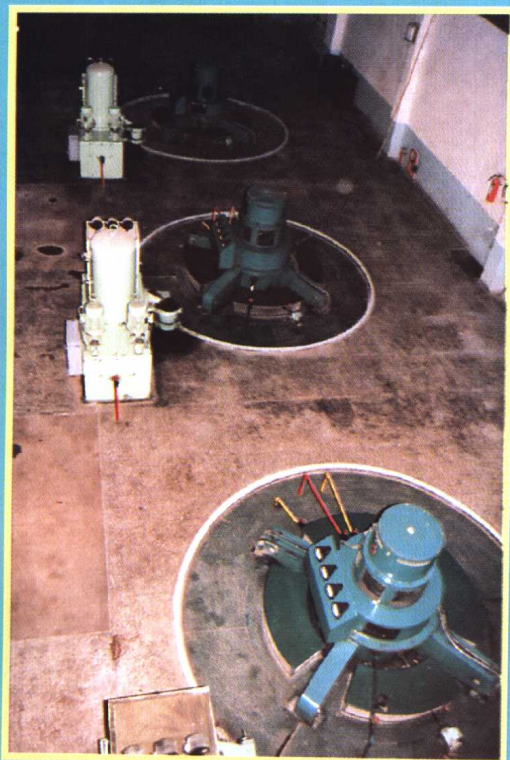
运行中的赤壁电站机组
