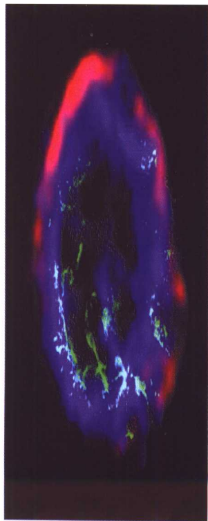
超新星残骸
