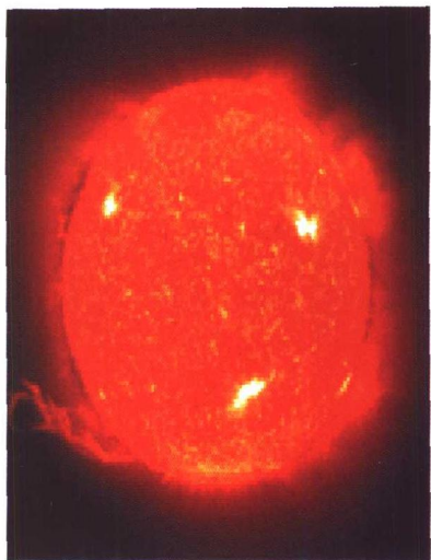
宇宙太阳系
