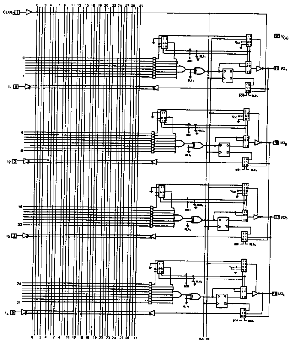
圖 C-9 PALCE16V8 之內部結構圖 (AMD 公司之 DATA BOOK)
