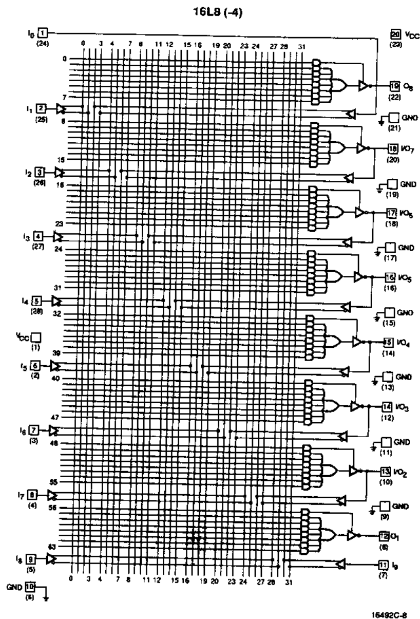
圖 C-7 PAL16L8 之內部結構圖 (AMD 公司之 DATA BOOK)
