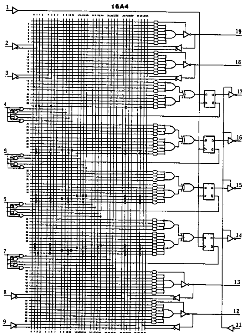
圖 C-3 PAL16A4 之內部結構圖 (AMD 公司之 DATA BOOK)
