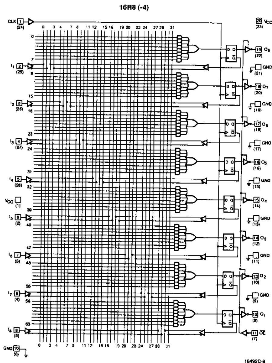
圖 C-8 PAL16R8 之內部結構圖 (AMD 公司之 DATA BOOK)
