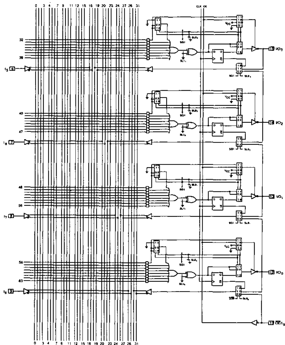
圖 C-10 PALCE16V8 之內部結構圖 (續)(AMD 公司之 DATA BOOK)
