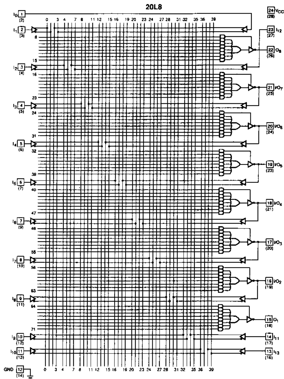
圖 C-11 PAL20L8 之內部結構圖 (AMD 公司之 DATA BOOK)
