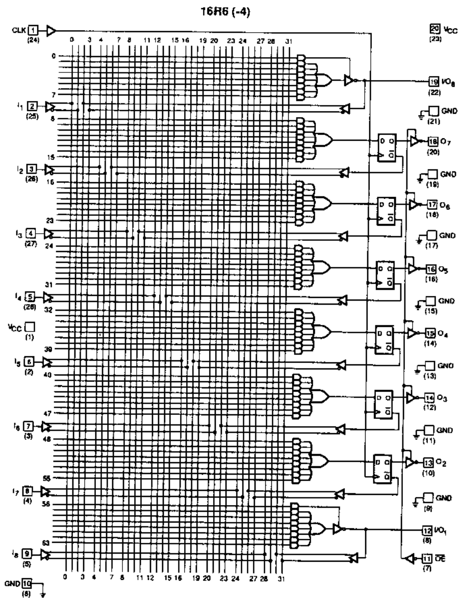
圖 C-5 PAL16R6 之內部結構圖 (AMD 公司之 DATA BOOK)
