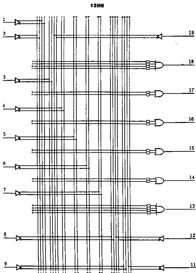
圖 C-1 PAL12H6 之內部結構圖 (AMD 公司之 DATA BOOK)
