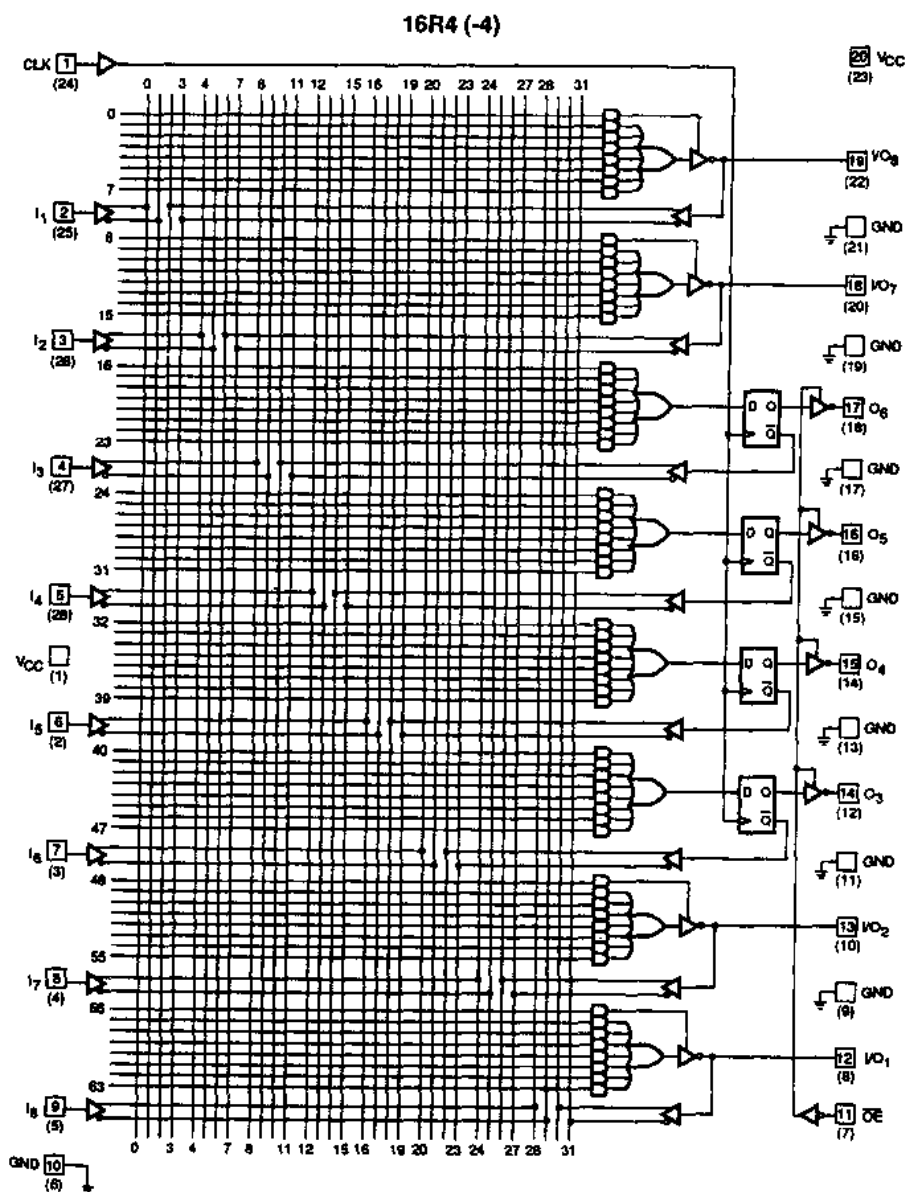
圖 C-6 PAL16R4 之內部結構圖 (AMD 公司之 DATA BOOK)
