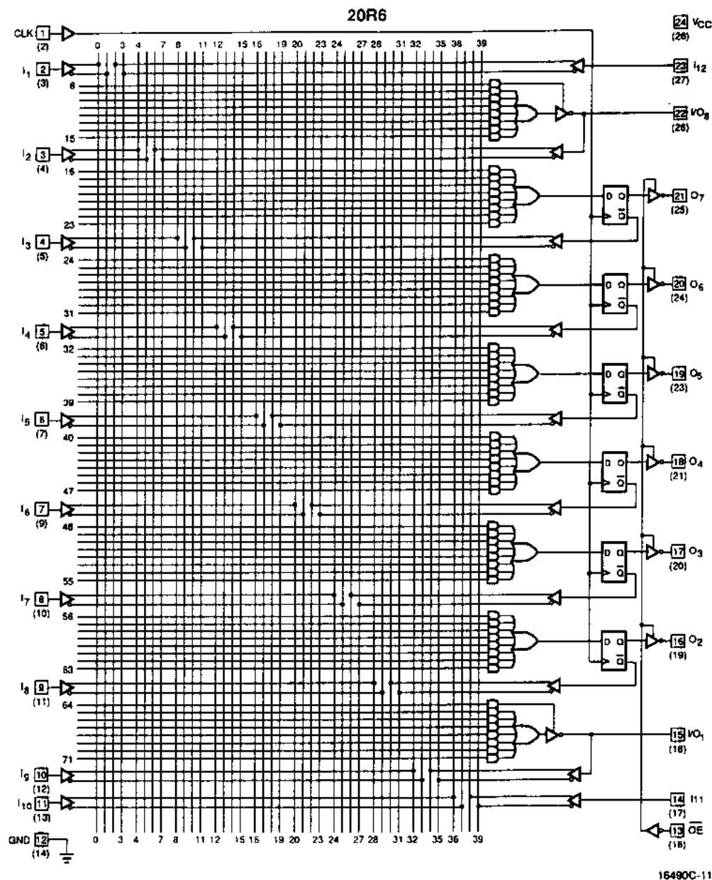
圖 C-13 PAL20R6 之內部結構圖 (AMD 公司之 DATA BOOK)
