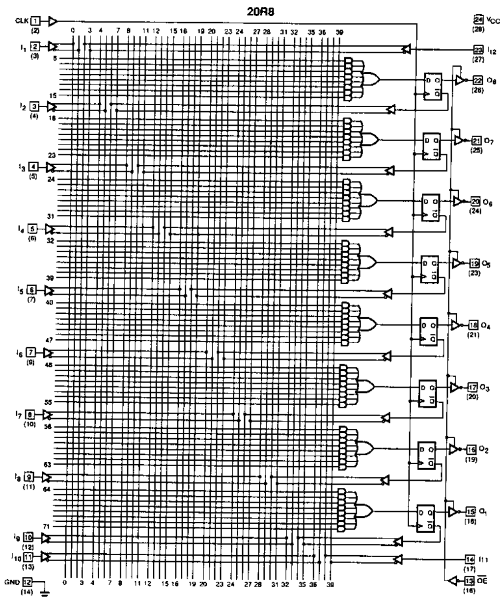
圖 C-12 PAL20R8 之內部結構圖 (AMD 公司之 DATA BOOK)
